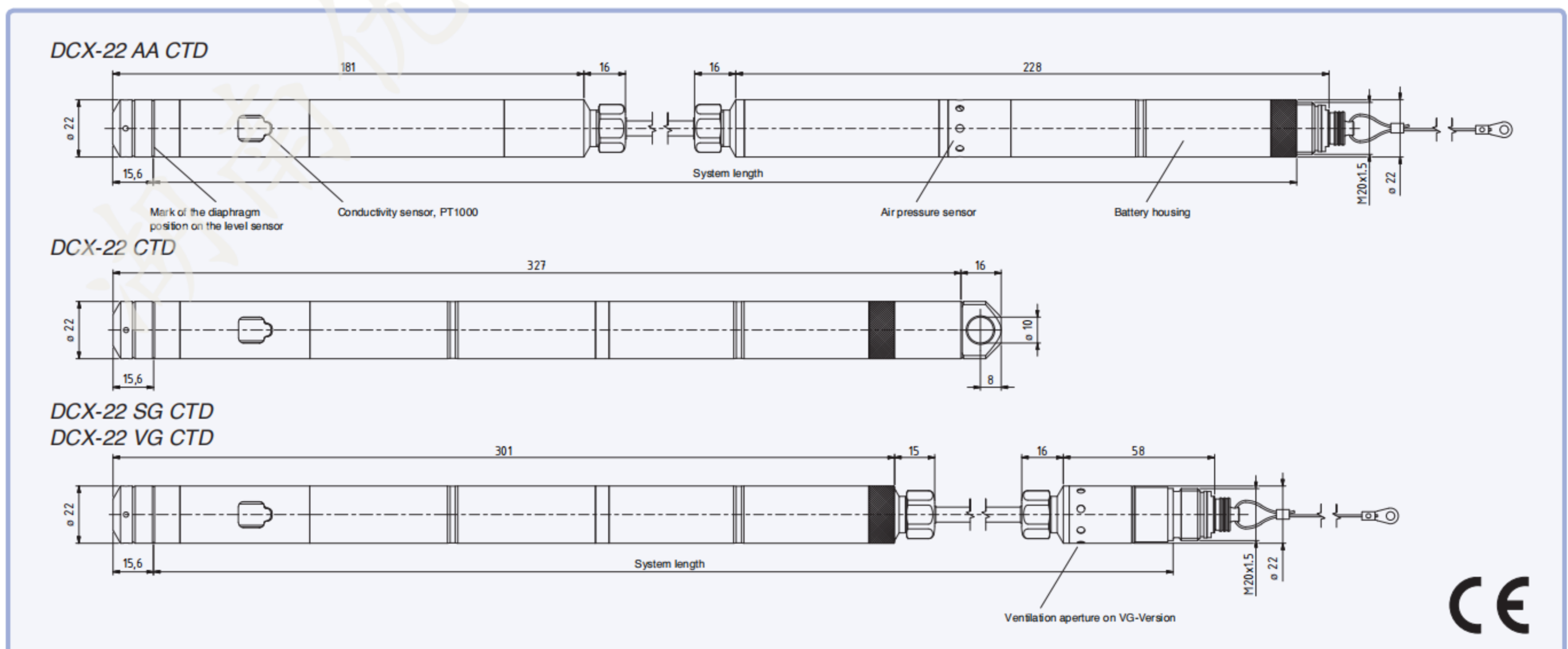
DCX-22 SG CTD DCX-22 VG CTD
